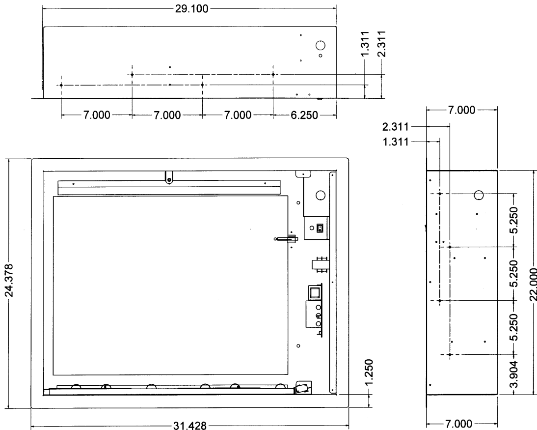
Fig. 7 — Dimensions
